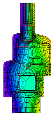
Isotermas
